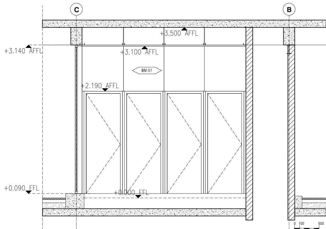
Elevation 01 (above) and elevation 03 (below) 立面01（上图）和立面02（下图）
