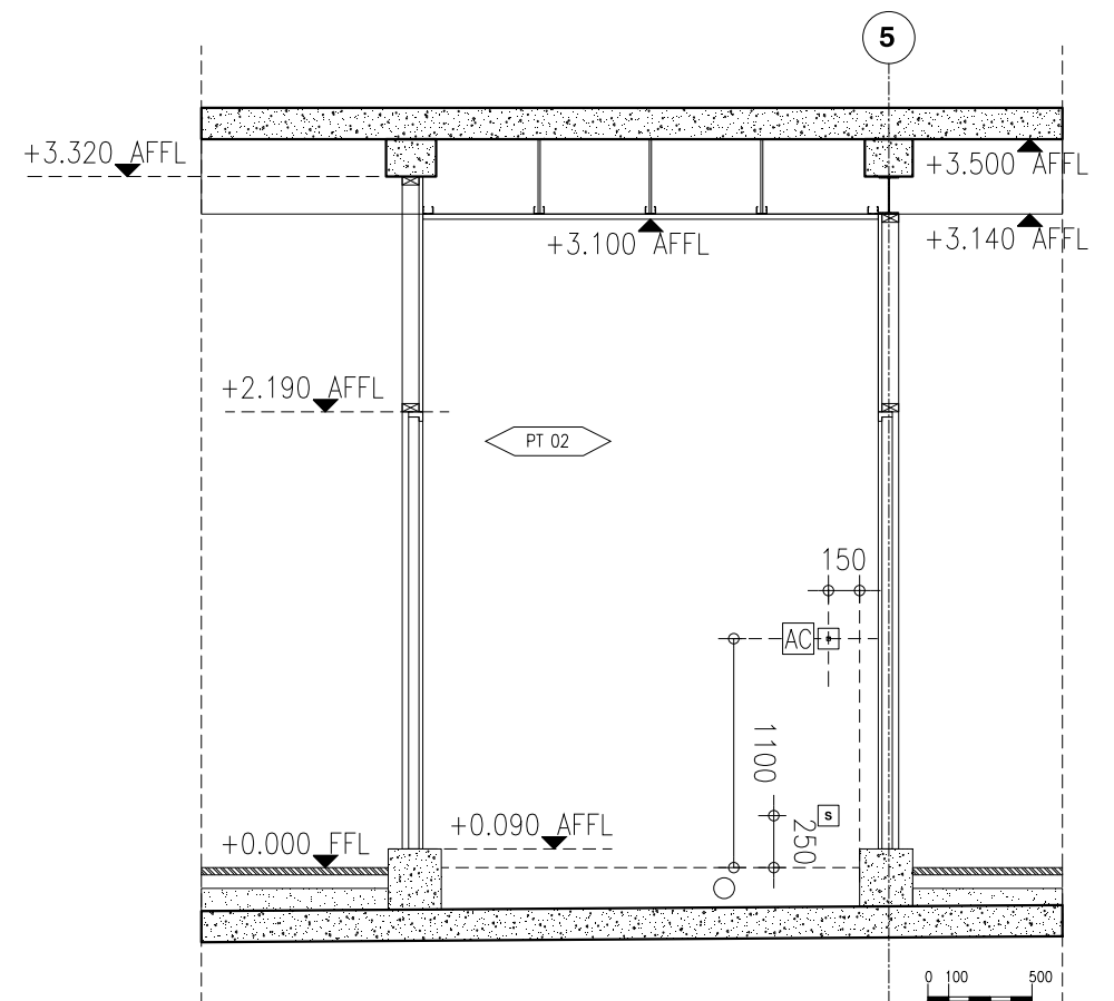
Elevation 02 (above) and elevation 04 (below) 立面02（上图）和立面04（下图）
